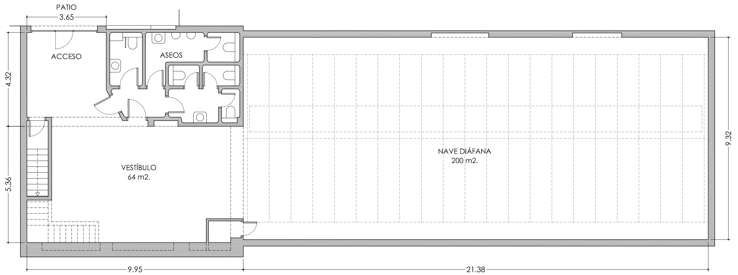
PLANTA
