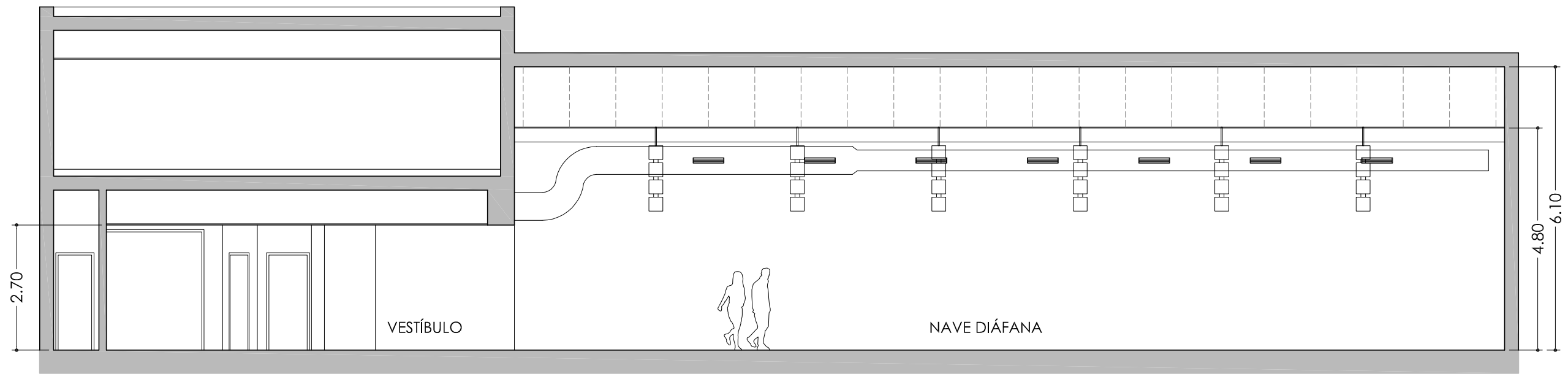
SECCIÓN
